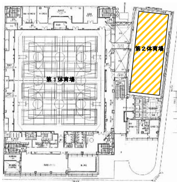
3 階平面図
